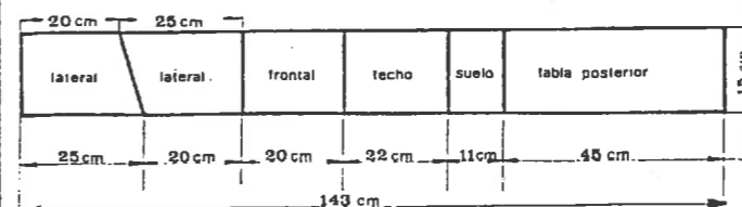
Caja nido para Carbonero, Herrerillo y Colirrojo.
